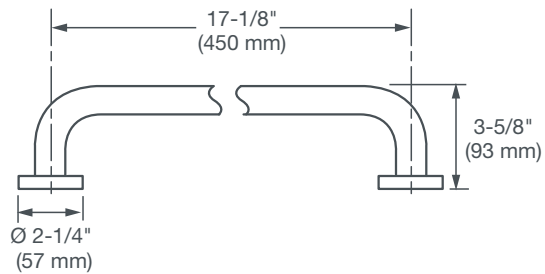
18" GRAB BAR
